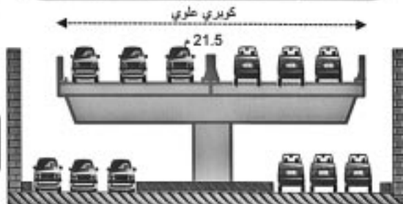
القطاع العرضي في حالة الكوبري
